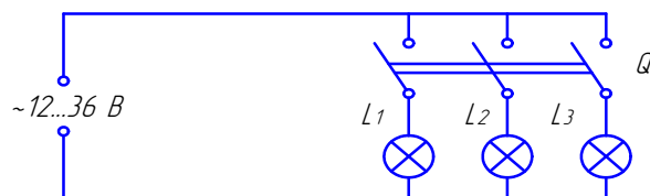
Рисунок 14 - Схема определение разновременности касания контактов КДВ
