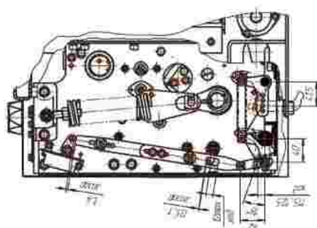
Рисунок А. 1 – Габаритные, присоединительные и установочные размеры вакуумного выключателя ВВУ-СЭЩ-П-10-25/1250 УЗ
