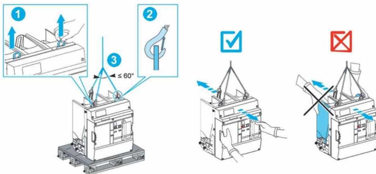
Рисунок 13 – Подъемно-транспортные операции
