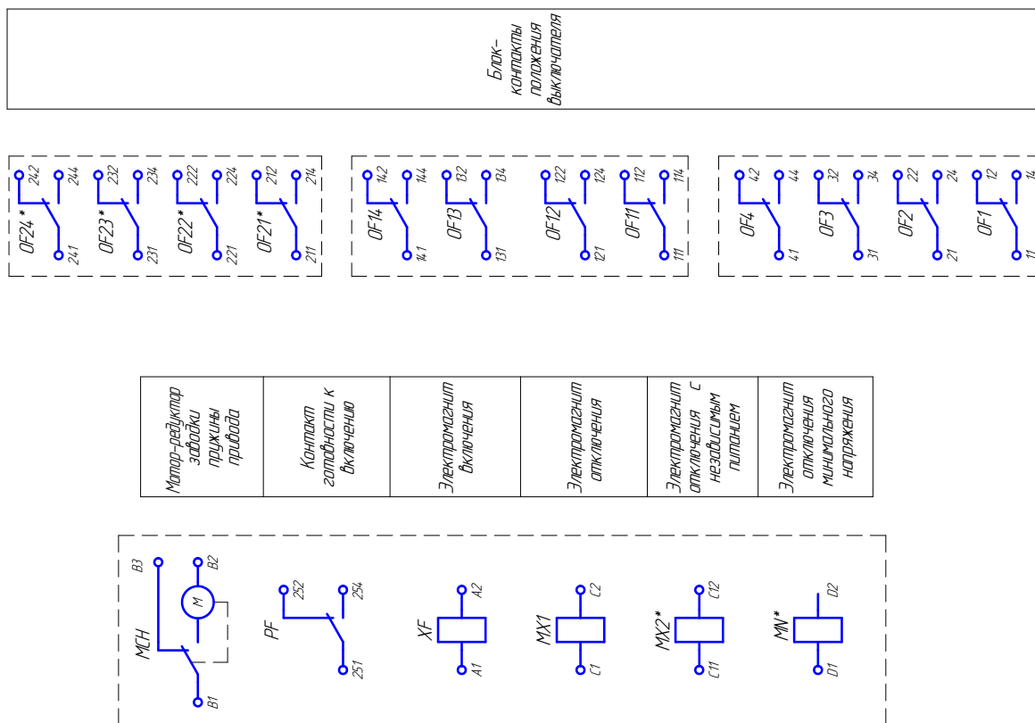
Рисунок Б.1 – Схема электрическая принципиальная вакуумных выключателей типа ВВЕ-СЭЩ-10
